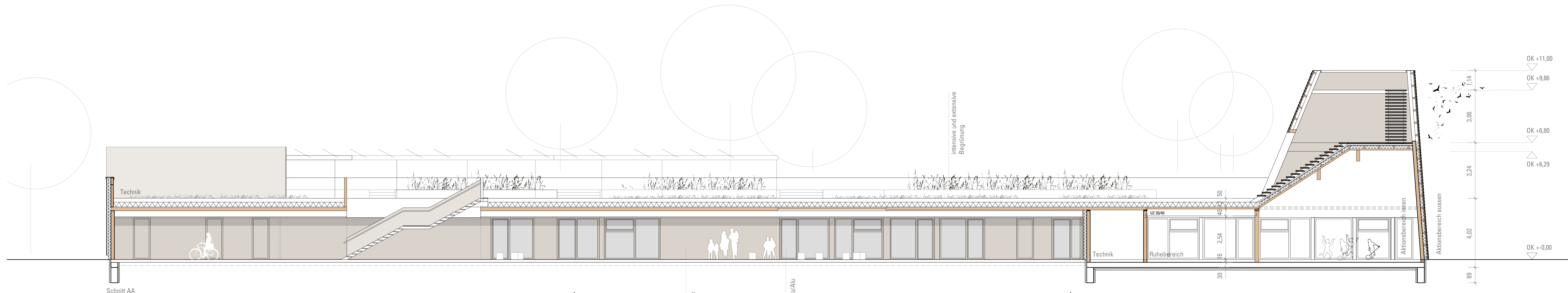
Schnitt AA
